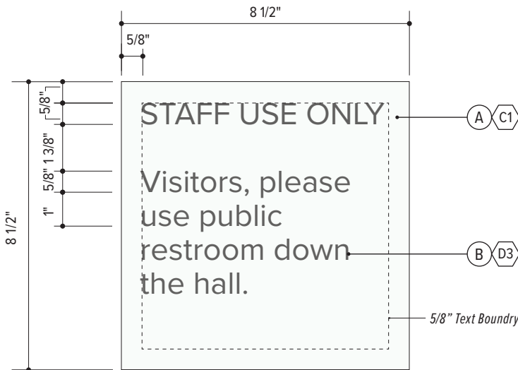
Front View Scale: 3"=1'-0"
