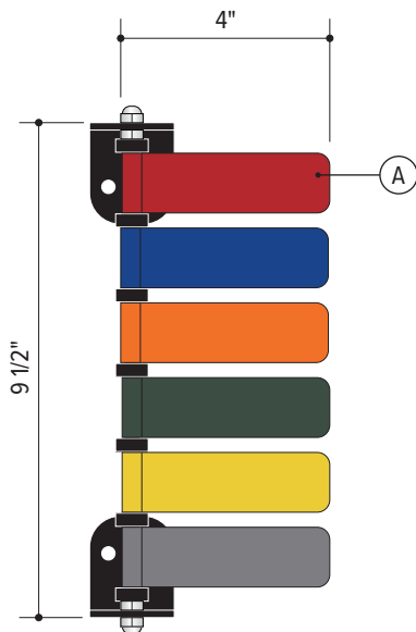
Front View Scale: 3"=1'-0"
