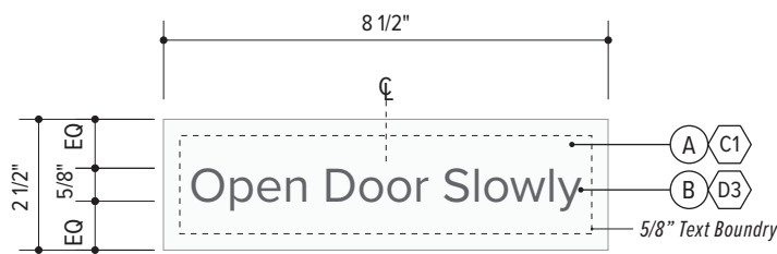
Front View Scale: 3"=1'-0"
